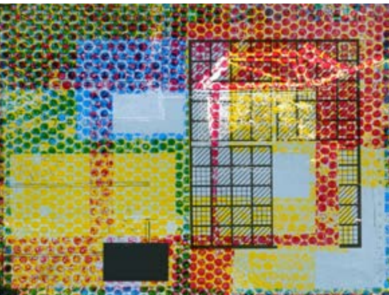
Demi-vies et le temps n° 1
