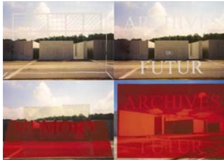
Un site archivé pour alpha, bêta, gamma
