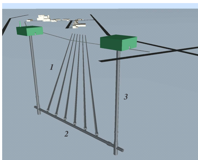
Figuur 3 – Het voorontwerp van diepe berging ontwikkeld door STOLA-Dessel, met de zes bergingsgalerijen (1), de hoofdgalerij (2) en de twee toegangsschachten (3) [figuur STOLA-Dessel].
