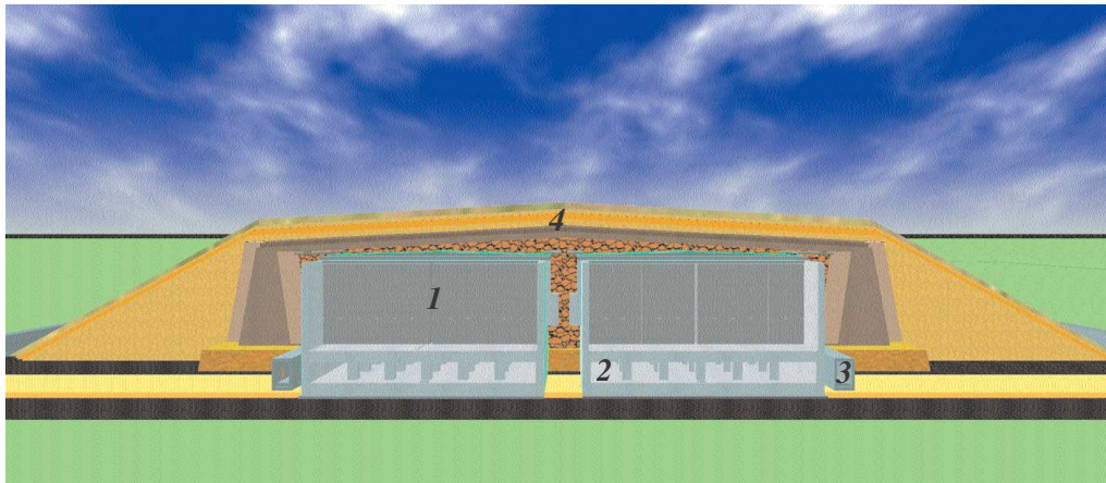
Figuur 2 – Het voorontwerp van oppervlakteberging ontwikkeld door STOLA-Dessel, met één van de twee dubbele rij modules (1), de kelderstructuur (2), de twee inspectiegalerijen (3) en de meerlagige afdeklaag (4) [figuur STOLA-Dessel].
